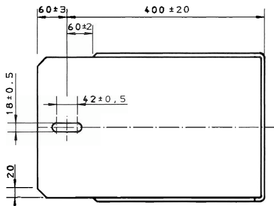
Schnitt A-A
