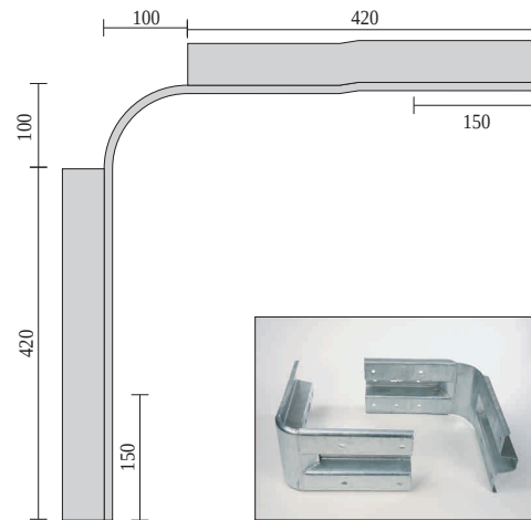
Best.-Nr. 5508, Eckstück B, innen 90°
