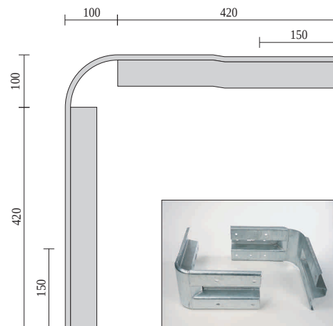
Best.-Nr. 5509, Eckstück B, außen 90°
