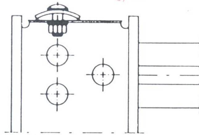
Schnitt B-B
