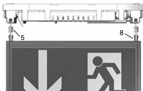
Baldachin-Querschnitt Canopy section
