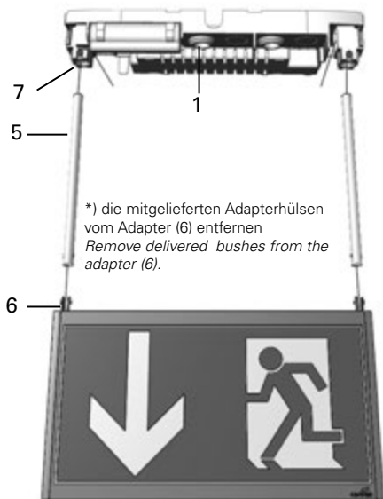
Baldachin-Querschnitt Canopy section
